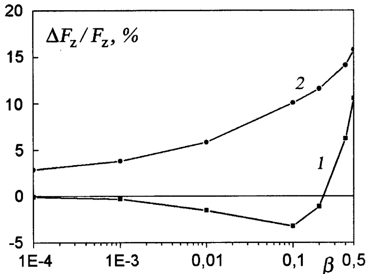
Рис. 11. Относительные отклонения приближенных формул для силы от значений, полученных методом изображений. Кривая 1 – значения, полученные по формуле (26) с использованием E_0 = (1 + 2/3\beta) < E_0 > , кривая 2 – значения, полученные по формуле (27)
