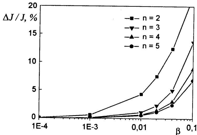
Рис. 13. Относительная ошибка вычисления значений интеграла J по приближенному выражению (33), по сравнению со значениями, полученными методом изображений ( m = 1000 )
