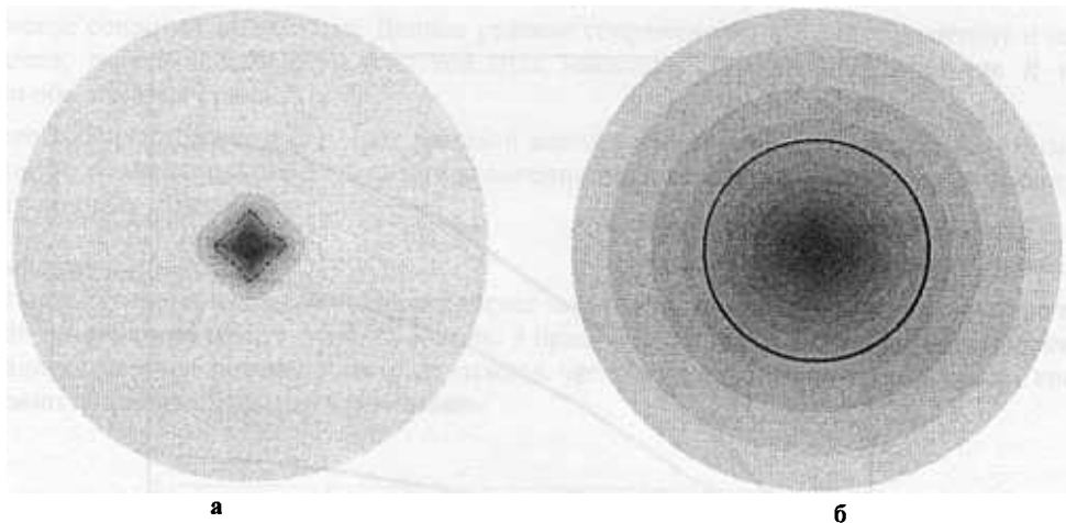
Рис. 6. Распределение температуры в окрестности тепловой трубы с четырьмя ребрами (ширина 10 см) на начальной (а, \Delta t = 1 сут) и промежуточной стадии процесса (б, \Delta t = 60 сут)
