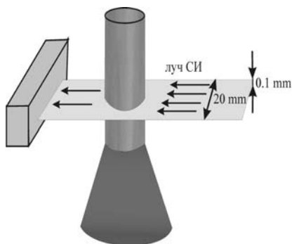
Рис. 17. Схема постановки экспериментов.
