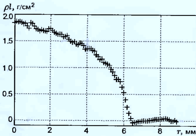
Рис. 5. Распределение количества просвеченного вещества по радиусу, восстановленное по калибровочной зависимости
