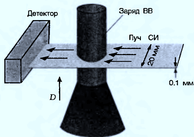
Рис. 1. Схема постановки экспериментов
