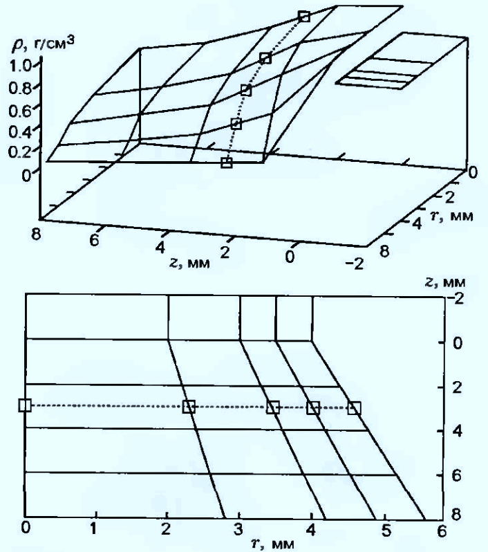
Рис. 7. Интерполяционная сетка для восстановления плотности:
