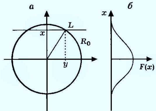
Рис. 3. Схема обработки результатов регистрации проходящего через образец излучения ( x, y — координаты вдоль и поперек луча)
