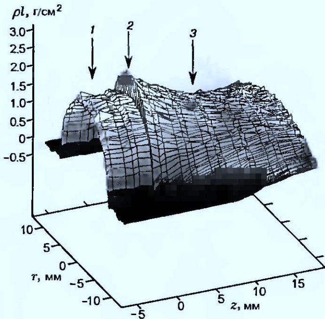
Рис. 6. Пространственное распределение количества просвеченного вещества:
