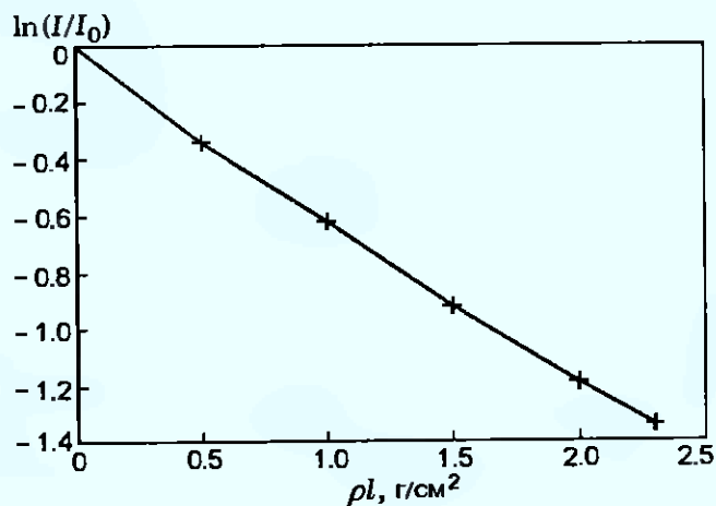
Рис. 4. Калибровочная зависимость для определения количества просвеченного вещества
