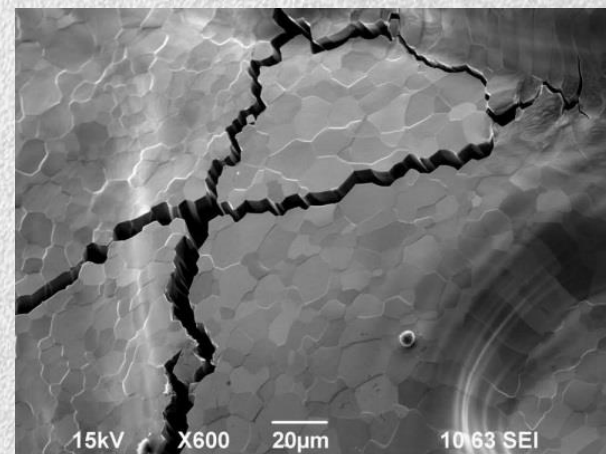
Трещина на вольфраме после импульсной плазменной нагрузки
