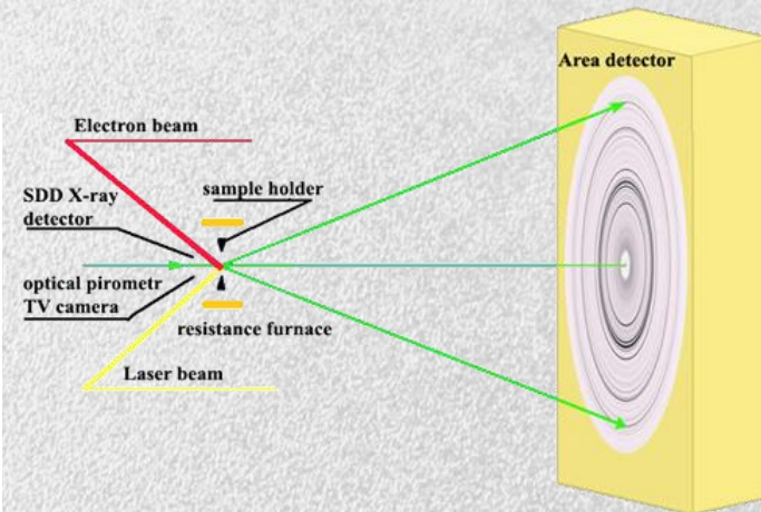
Схема эксперимента
