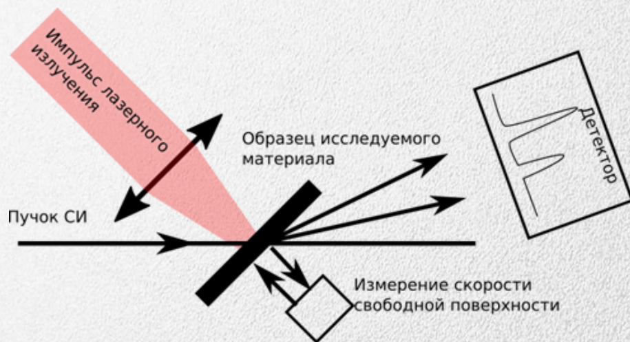
Схема эксперимента
