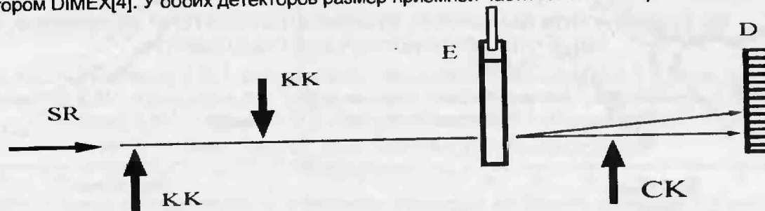
Рис. 1. Схема постановки экспериментов по измерению МУРР
