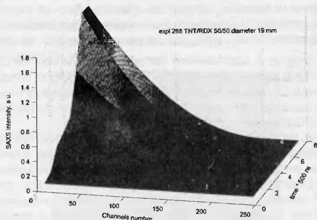
Рис. 4. Поведение МУРР после прохождения детонационного фронта
